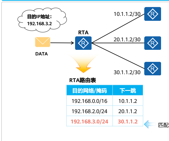
最长匹配示例
