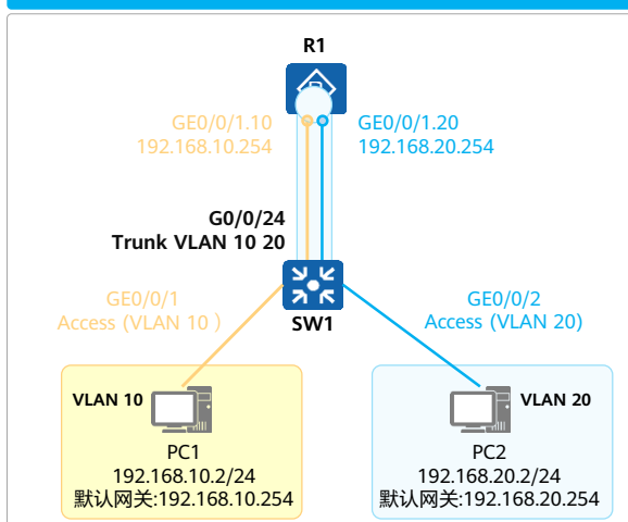
物理连接图
