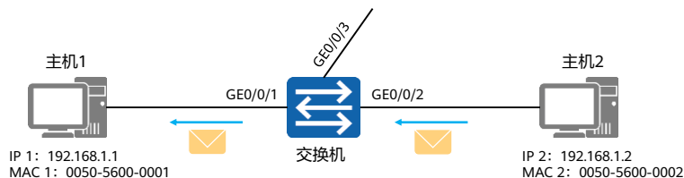
交换机的MAC地址表
