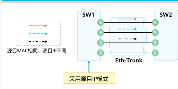
合适的负载分担算法
