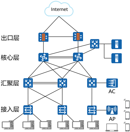
某外贸公司网络拓扑
