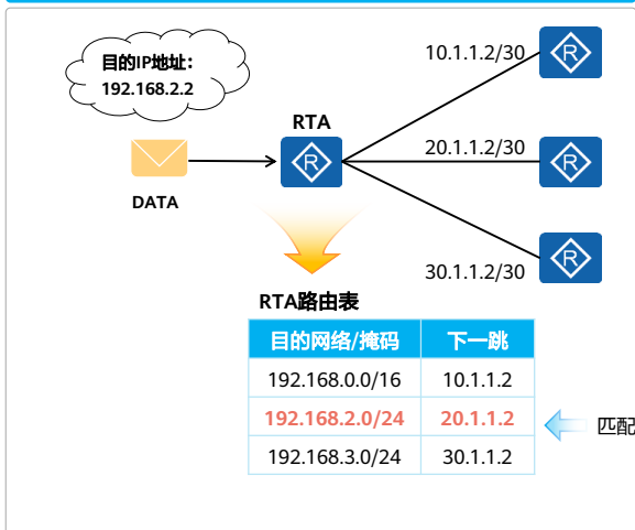
最长匹配示例
