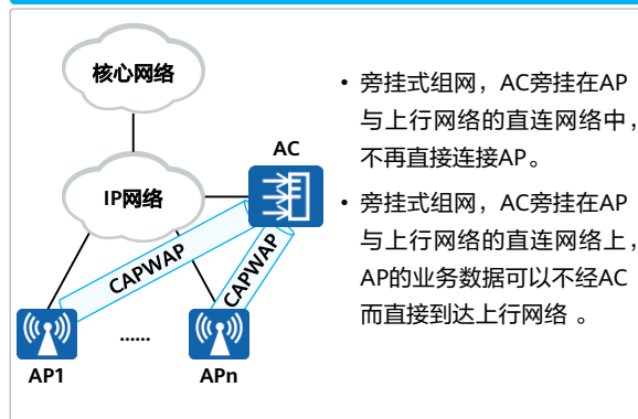
旁挂式组网
