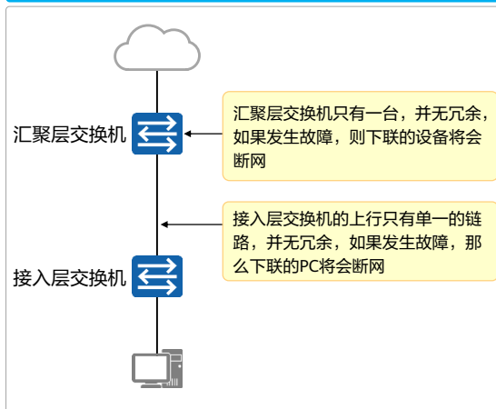
一个缺乏冗余性设计的网络
