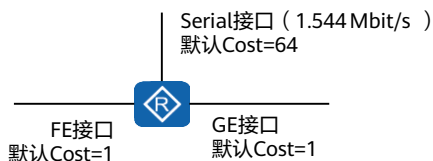
OSPF接口Cost值
