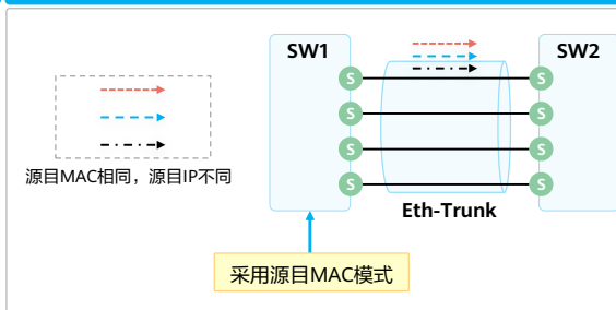
不合适的负载分担算法
