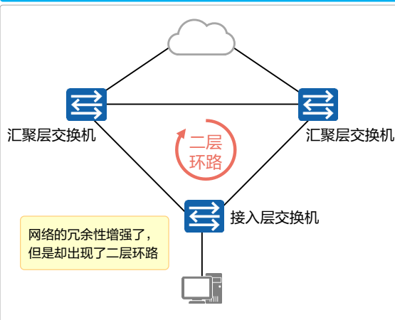
引入冗余性的同时也引入了二层环路
